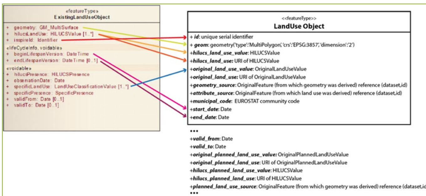
Obrázek 22: Přejechod od INSPIRE modelu prvku využití půdy k modelu OLU.
