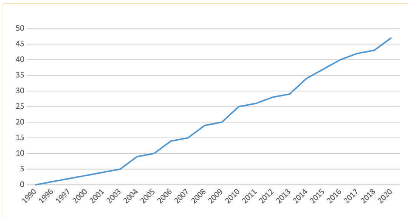
Graf 2. Vývoj počtu rezistentních druhů plevelů rezistentních vůči účinné látce glyfosát (Upraveno dle Ian Heap, Weedsience. Org. 2019)
